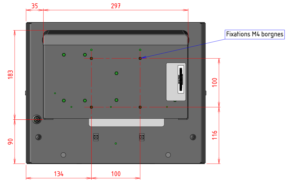
VUE ARRIERE
